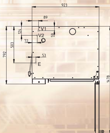
TABULKA TECHNICKÝCH PARAMETRŮ 10 x GN1/1
